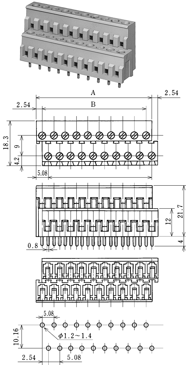
プリント基板寸法 PCB specifications
