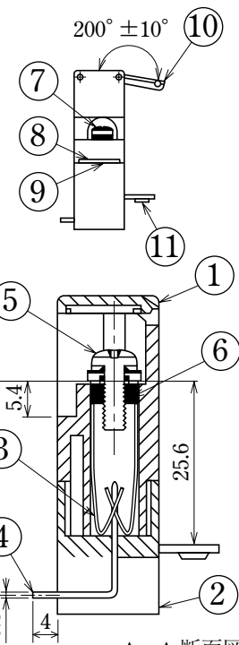
A-A 断面図 A-A sections
