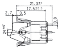
ボックスには端子番号を表示していません。 Terminal number not shown on box.
