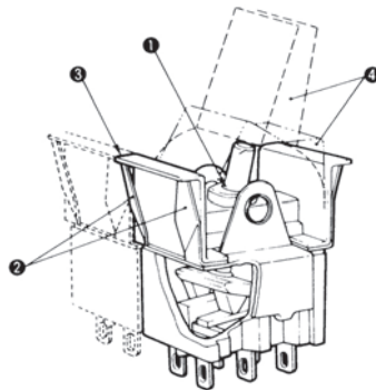
定格表示側 Rating marking side
